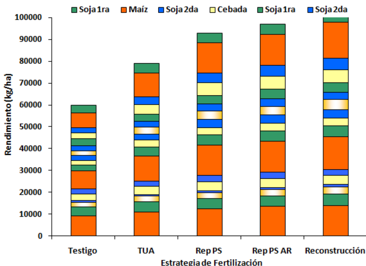
Figura 1. Producción por cultivo ( \text{kg ha}^{-1} ) de diferentes estrategias de fertilización acumulada en una secuencia maíz - soja - trigo/soja - cebada/soja - maíz - soja - cebada/soja - trigo/soja - soja - cebada/soja - maíz. Arribeños, General Arenales. Campañas 2006/07 a 2017/18.
