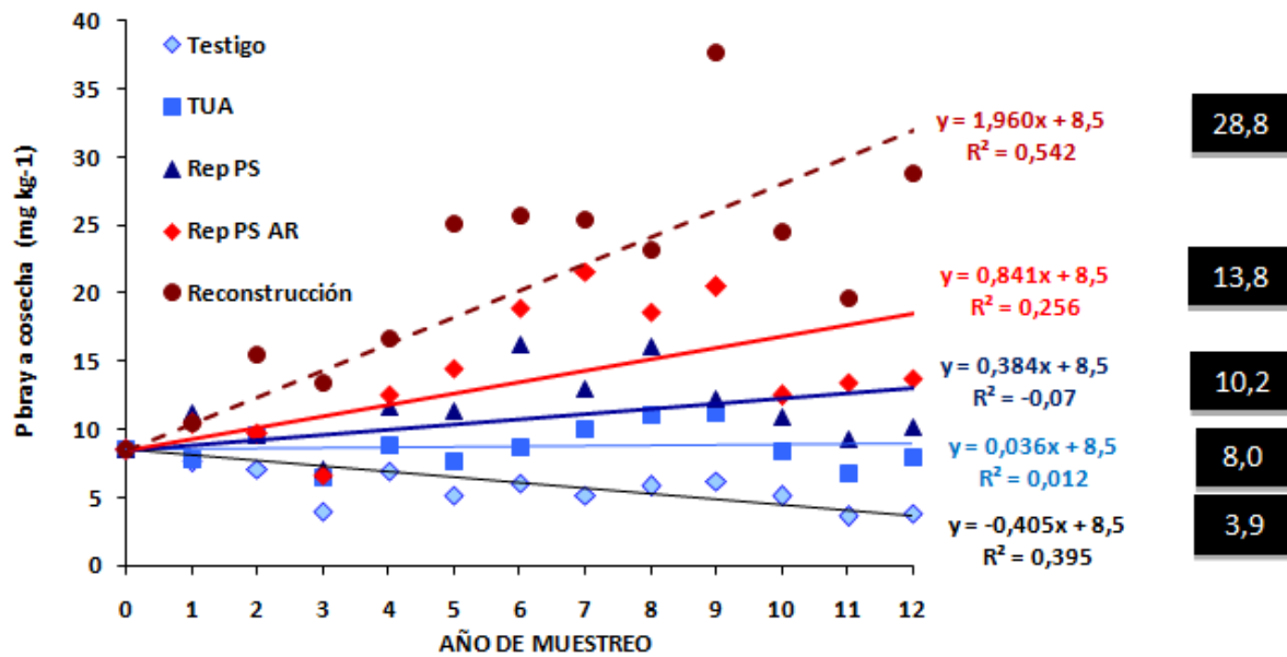
Figura 2. Evolución del P extractable en suelo (Bray-1, 0-20 cm) según estrategia de fertilización, luego de doce campañas y diecisiete cultivos, hasta la campaña 2017/18. A la derecha se indica el último valor determinado, en julio 2018.
