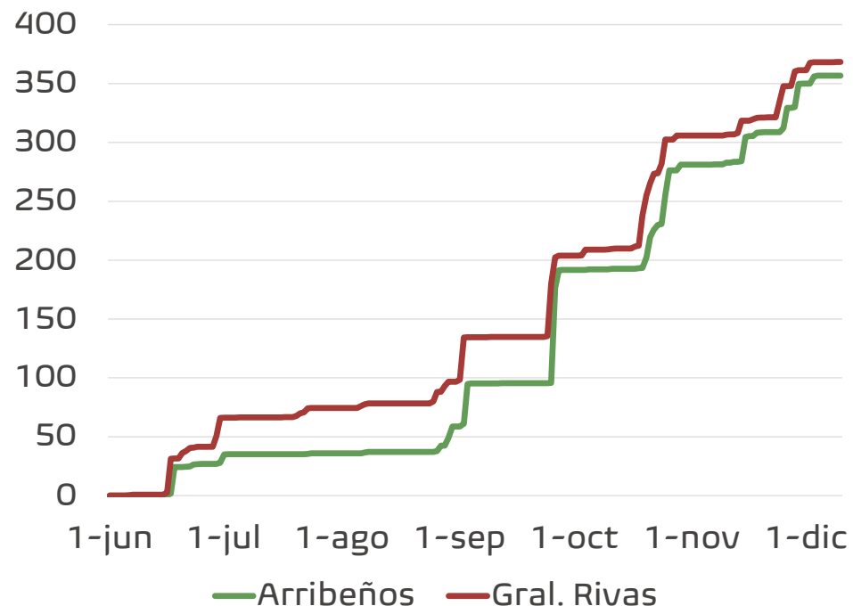
Precipitación acumulada (mm)
