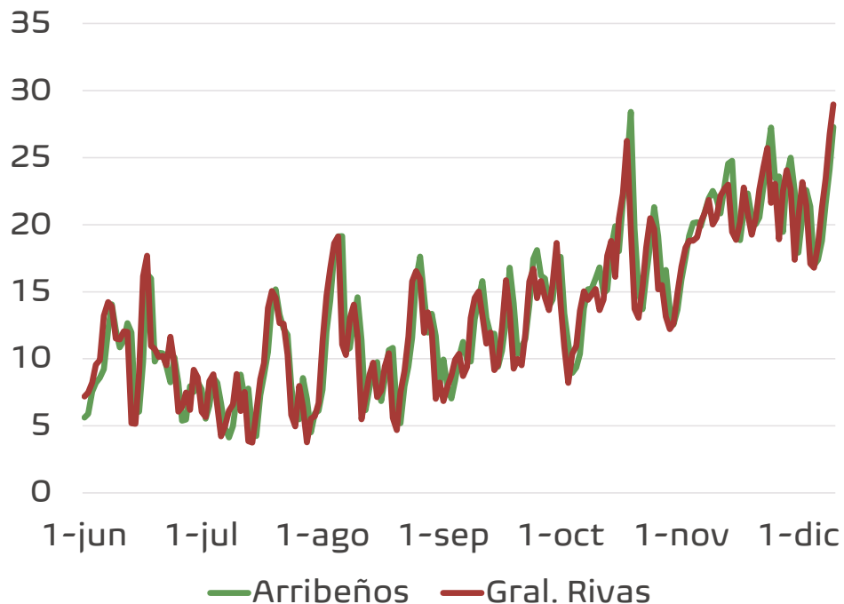
Temperatura media (°C)
