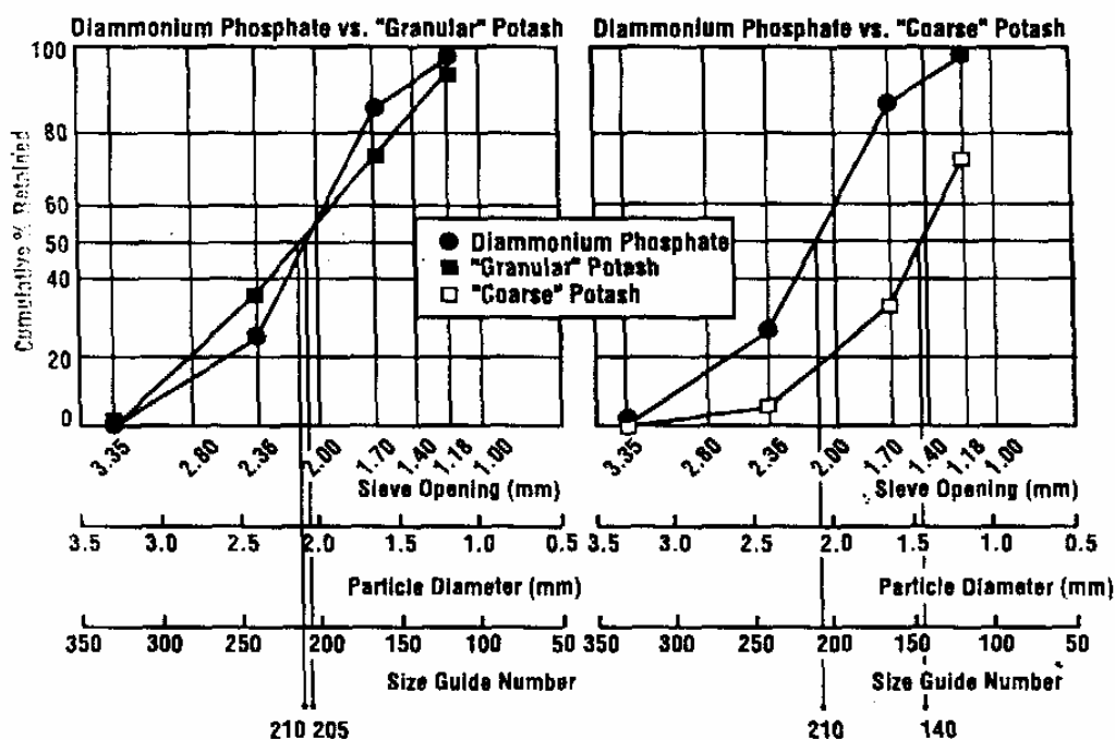
Figura 3 Evaluación de compatibilidad física de ingredientes de mezclas físicas de acuerdo a la acumulación de distribución de tamaños de partículas y uso del SGN (Fertilizer Manual, 1998).
