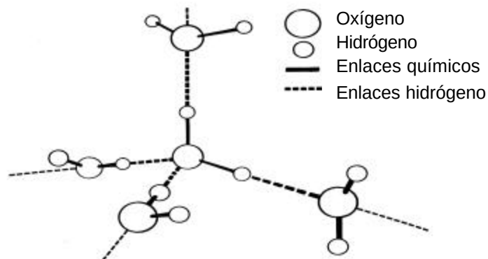
Figura 1-2. Los "puentes" hidrógeno ("enlaces", líneas punteadas) hidrógeno encadenan cada átomo de oxígeno que aparece en la estructura de cualquier molécula de agua con otras cuatro moléculas de agua ; dos de estos "puentes" involucran la participación de átomos de hidrógeno de una molécula dada de agua y las otros dos involucran la participación de átomos de hidrógeno provenientes de otras moléculas de agua. La energía de tales enlaces de hidrógeno es intermedia entre la energía de los enlaces químicos usuales que existen entre átomos de una dada molécula (líneas sólidas) y la energía de la atracción molecular entre moléculas vecinas. La forma de estructura que aquí se muestra es la disposición geométrica de los átomos que se encuentran en el hielo ordinario. (Fuente: Scientific American 223(5):52-64, 69-71).
