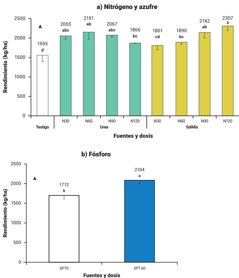
Figura 1. Rendimiento de Camelina sativa según fuente y dosis de fertilizante agregado. A) Nitrógeno – azufre. b) Fósforo. Letras distintas sobre las columnas representan diferencias significativas entre tratamientos (LSD \alpha=0,05 ), INTA Pergamino, año 2023.
