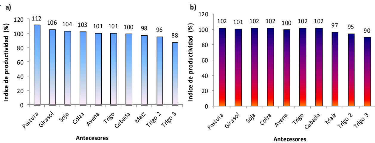
Figura 8. Efecto del cultivo antecesor sobre el rendimiento relativo de trigo sin nitrógeno (a) y con 46 kg.ha-1 de nitrógeno (b). Fuente: Ensayo rotaciones con labranzas. Chacra Experimental Integrada Barrow.
