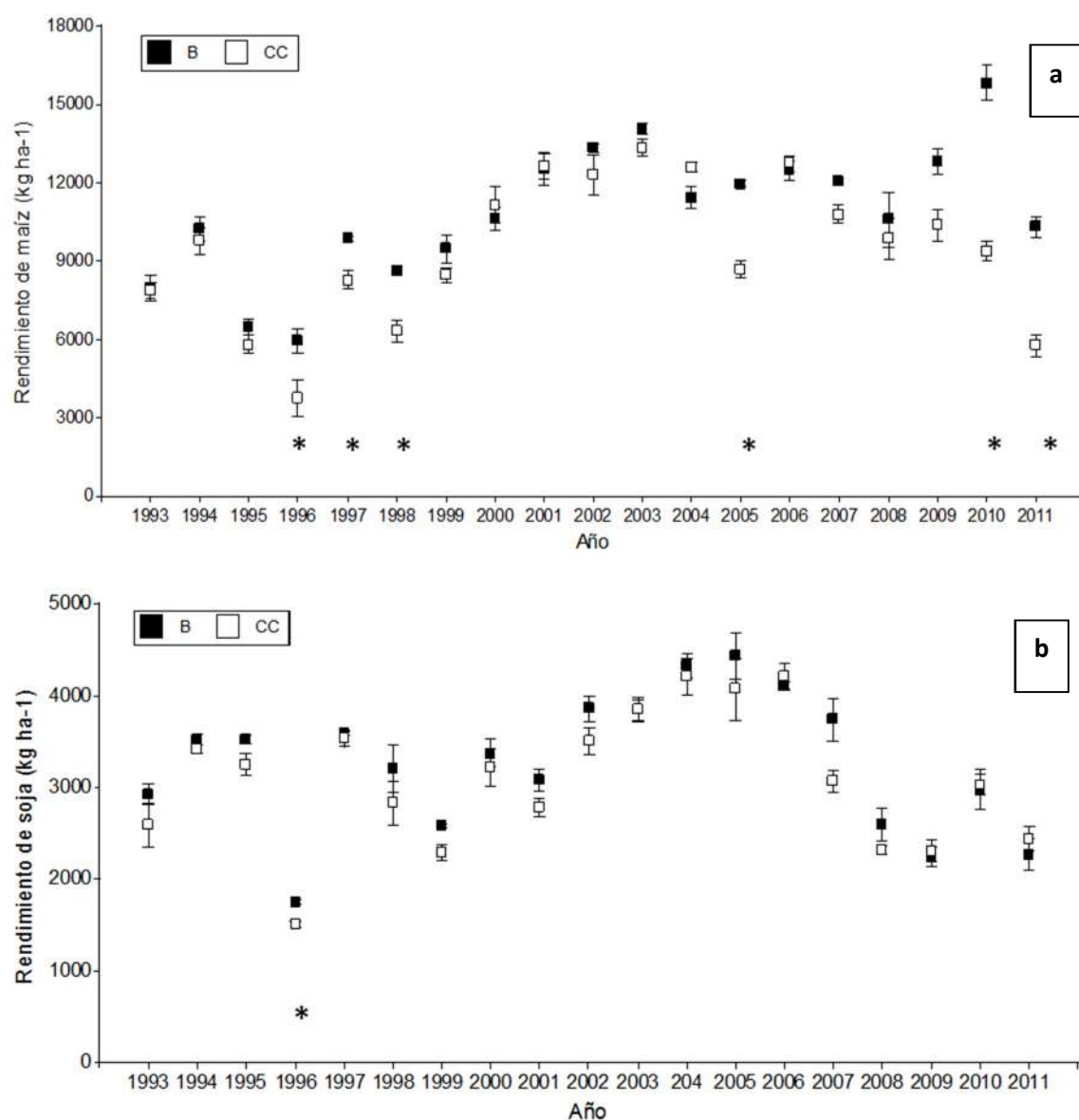
Figura 5: Rendimientos de maíz (a) y soja 1ra (b) en los tratamientos barbecho (B) y cultivos de cobertura (CC). Asteriscos indican diferencias significativas entre tratamientos. ( p < 0,05 ).
