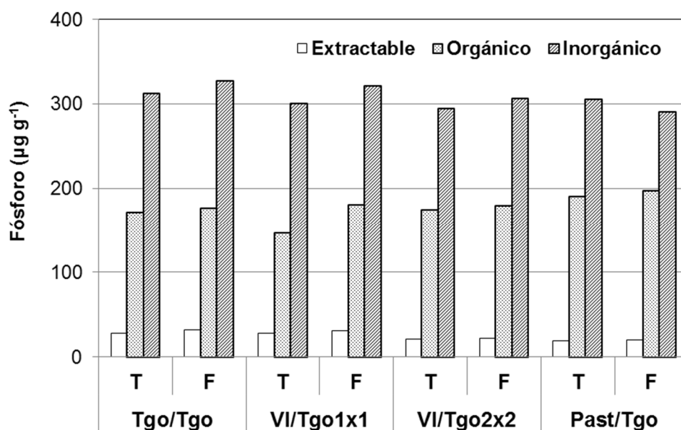
Figura 9 - Contenido de fósforo extractable, orgánico e inorgánico (capa 0-20 cm), luego de 27 años de tratamientos para el monocultivo (Tgo/Tgo), alternancia de verdeos anuales de invierno consociados con vicia (VI/Tgo1x1 y 2x2), y secuencia pastura-agricultura (Past/Tgo). T=testigo, F=fertilizado. Adaptado de Minoldo (2010)
